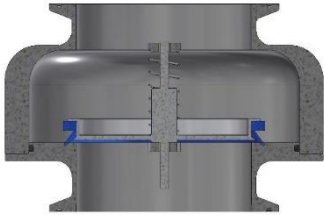
Überdruckventil im Ruhezustand, geschlossen .
