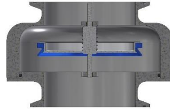
Überdruckventil bei Aktivierung, geöffnet .
